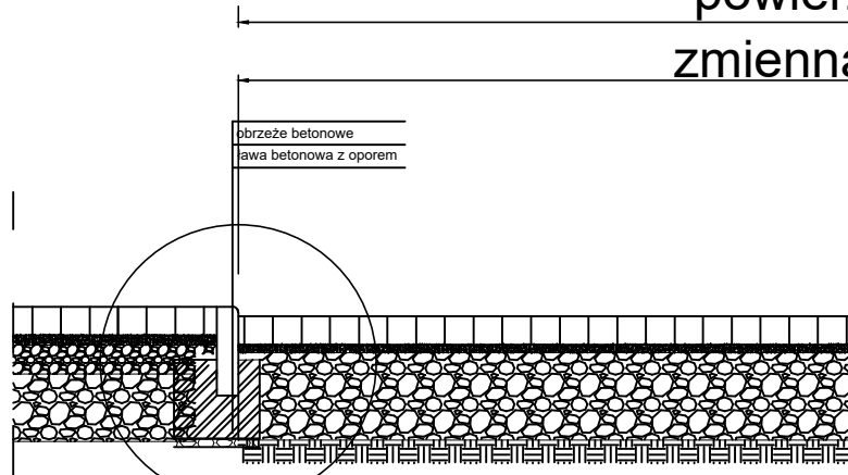
SZCZEGÓŁ B
