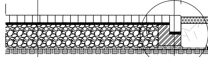
SZCZEGÓŁ A
