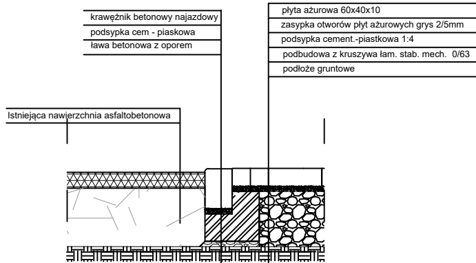
SZCZEGÓŁ A
