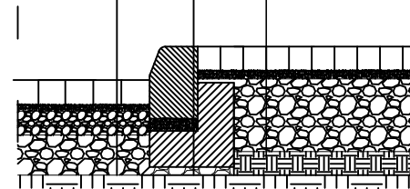
SZCZEGÓŁ B
